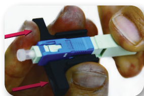
2- Destrave a fibra
