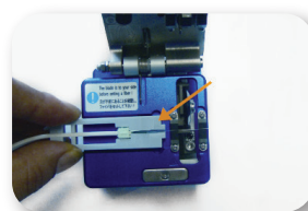
7- Encaixe e alinhe até o final
