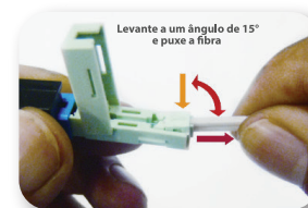
4- Puxe a fibra
