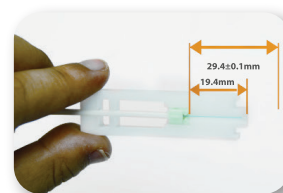
8- Especificação do comprimento da fibra
