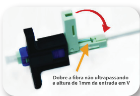
3- Complete a inserção da fibra
